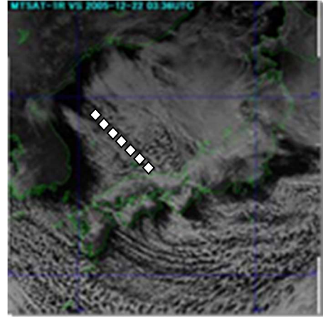
図4 気象衛星画像(可視)
