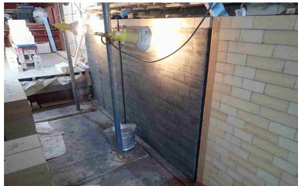
【写真④】耐火煉瓦施工（焼却炉）
