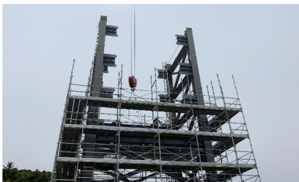
【写真①】煙突部鉄骨組立状況
